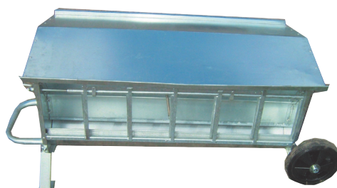
GUTTORM Gullsøya Kort kraftfôrautomat for lam på 120 cm. Med 12 eteplasser med justerbar halsåpning.
