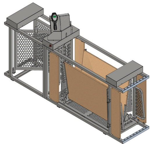
BioControl WSS3000 elektronisk vekt med sortering og elektronisk ID.
